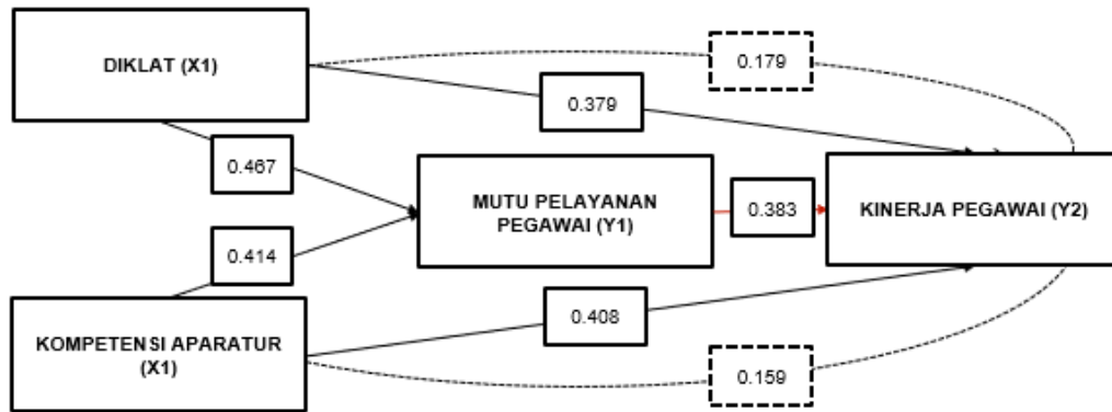
Gambar 2. Analisis Jalur
