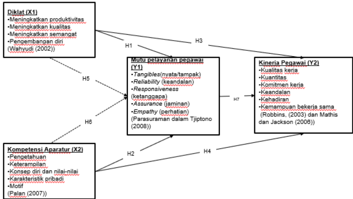
Gambar 1. Kerangka Pemikiran
